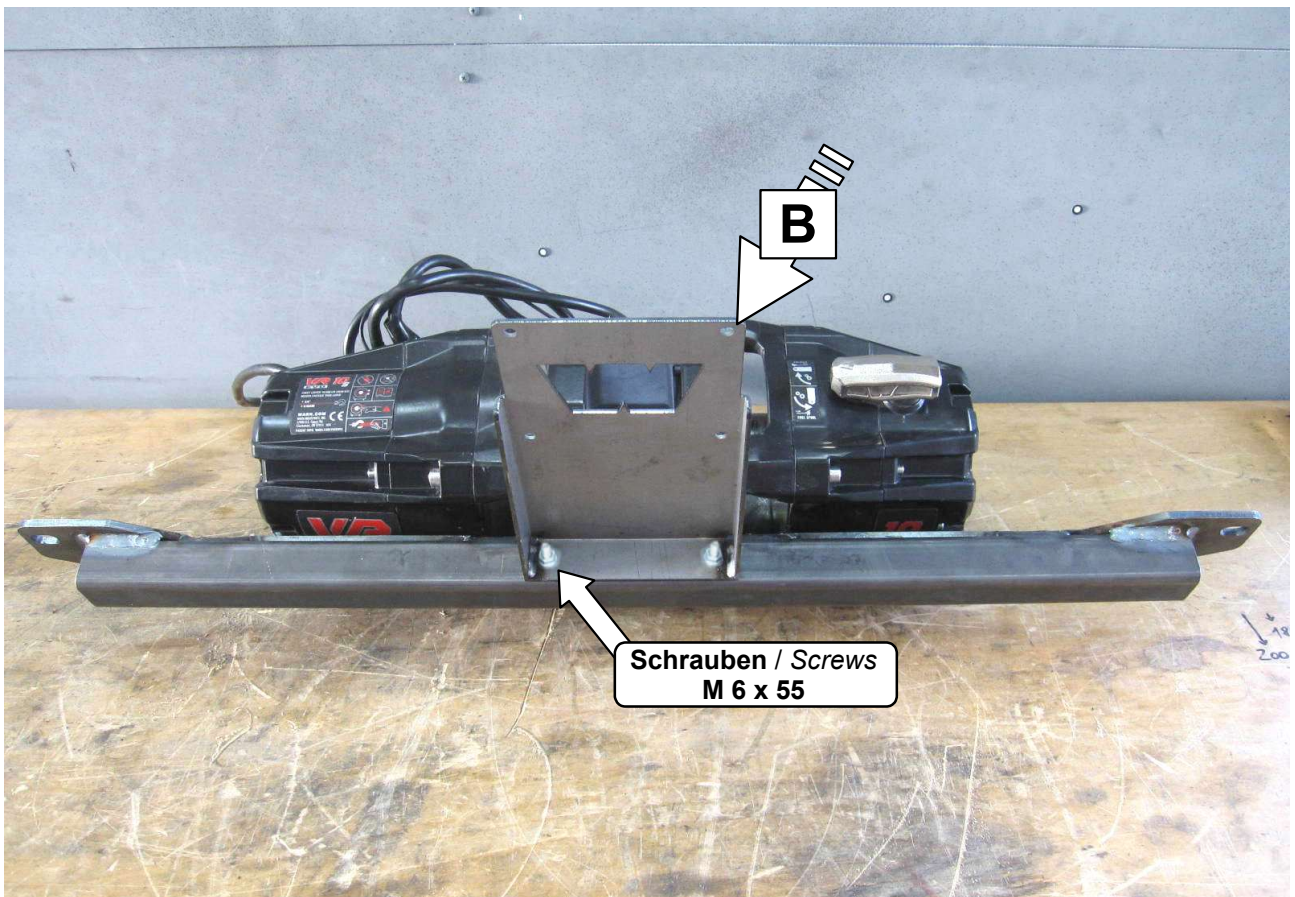
11 Schaltkastenhalter montieren! / Mount the bracket for switch box!
