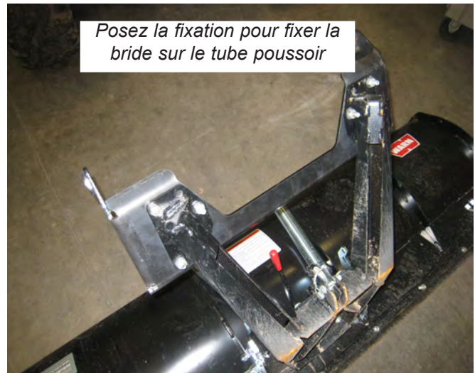
Figure 5 Installez les fixations
